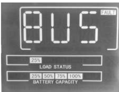
Рисунок 2-9. Сбой напряжения на шине постоянного тока
