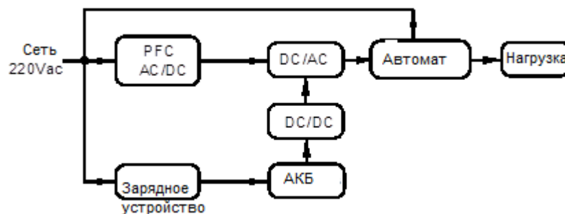
Рисунок 2.-7 Принципиальная схема работы ИБП
