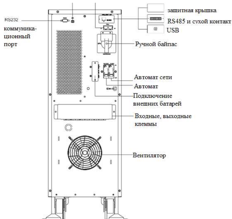
Рисунок 2-4. Задняя панель ИБП АБ-КР 11 Т 6 кВА/ 10 кВА
