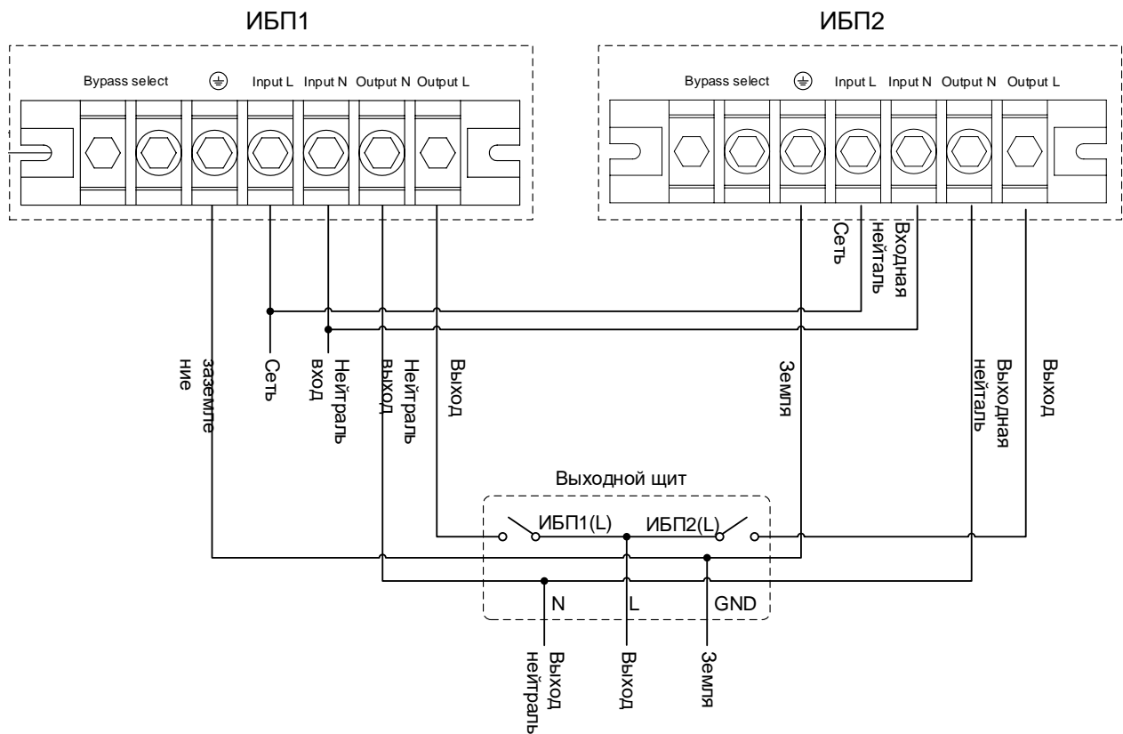
Рис 3.10 Схема подключения для ИБП 6кВА/ 10кВА при работе в параллель
