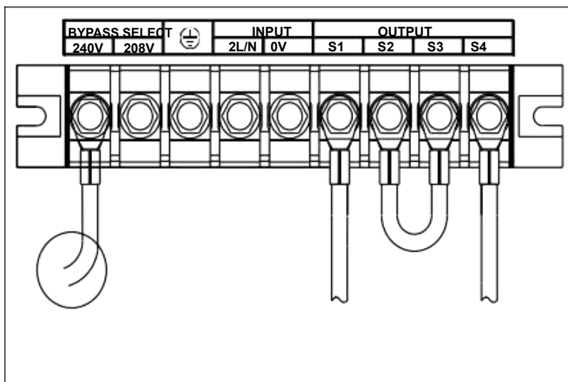
Рисунок3-4. Подключение кабелей.
