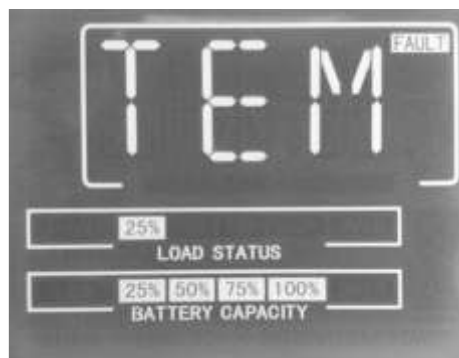
Рисунок 2-12. Перегрев IGBT
