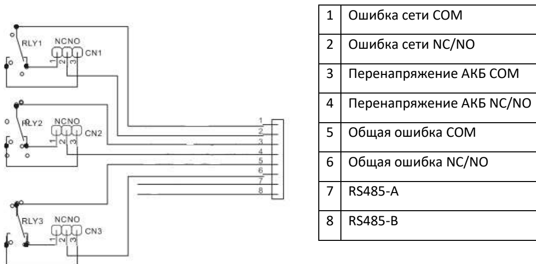
Рисунок 2-6. Назначение контактов порта RS485 и сухие контакты
